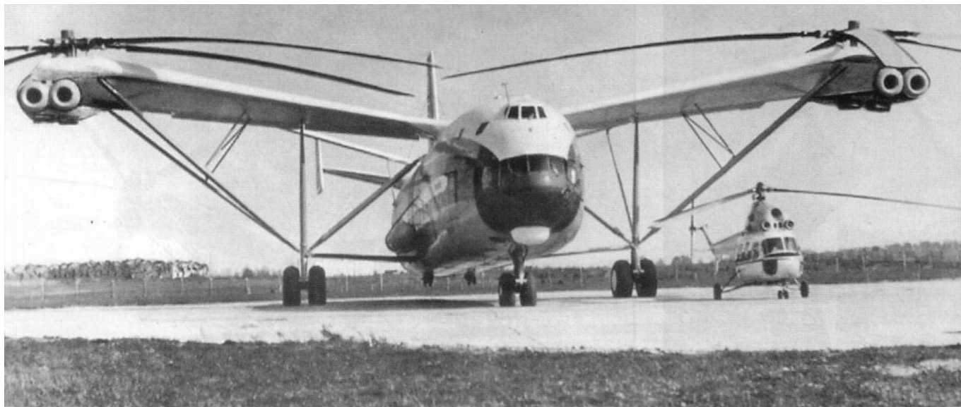
Ми-12, Московский вертолетный завод им. М. Л. Миля 12 © Wikimedia Commons - CC-by-3.0
